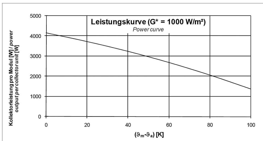
Kurve für AS 6 Großflächenkollektor
